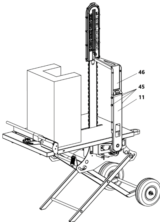
Рисунок 10 Общий вид станка с вырезанным U-блоков 11 – стойка; 45 – болт; 46 – кронштейн
