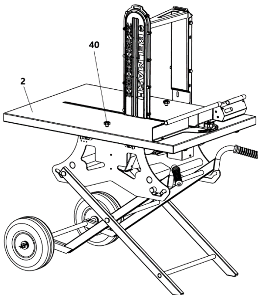
Рисунок 13 Общий вид станка в транспортном положении
