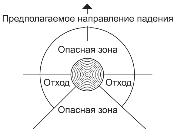
Рисунок 11 — Опасная зона при валке дерева
